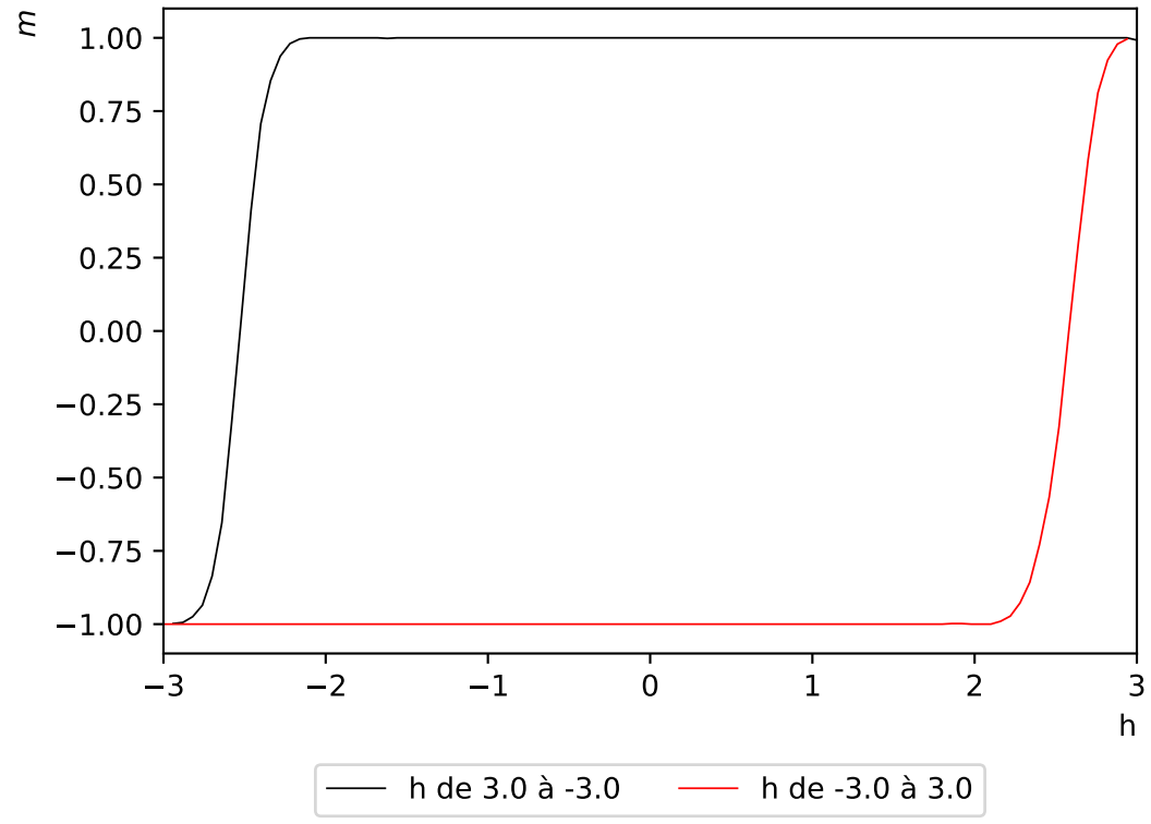
Hystérésis de l'aimantation - réseau de taille L=32 - champ magnétique d'amplitude h=3 à T=0.5
